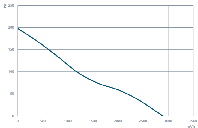
AXIP 400-5-25
