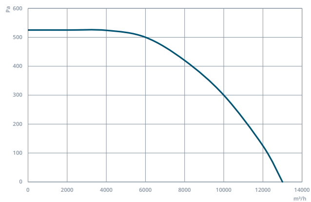
HMEF 710
