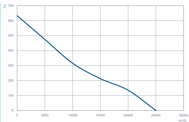
CAXIDIK 800-5-35
