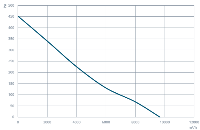
CAXIDIK 630-5-30
