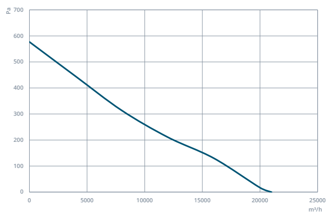
CAXIDIK 800-5-30
