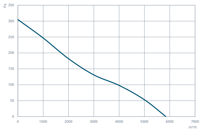
AXIP 500-5-25
