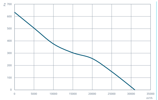
DAXI 800-5-35
