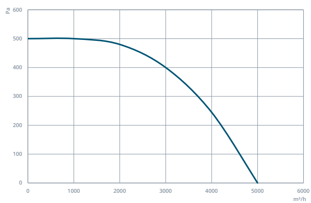
DRAD 450
