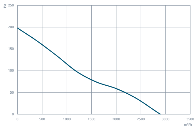
HAXI 400-5-25
