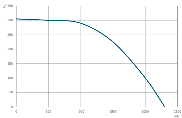
DRAD 355
