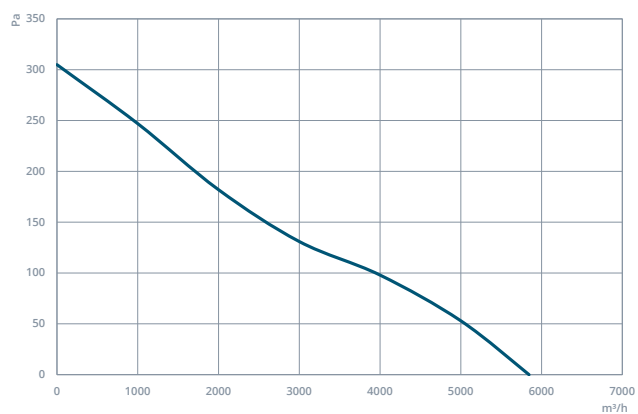
HAXI 500-5-25
