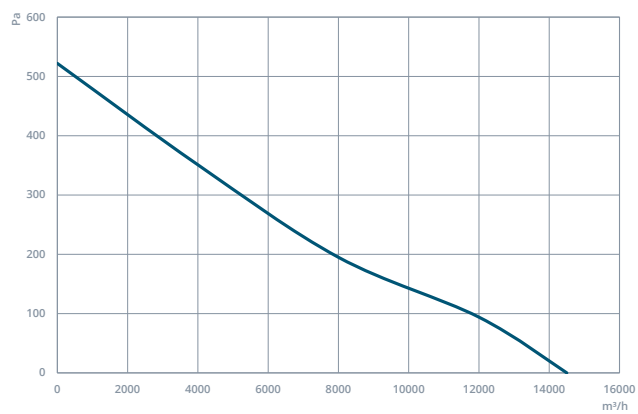
CAXIDIK 710-5-30
