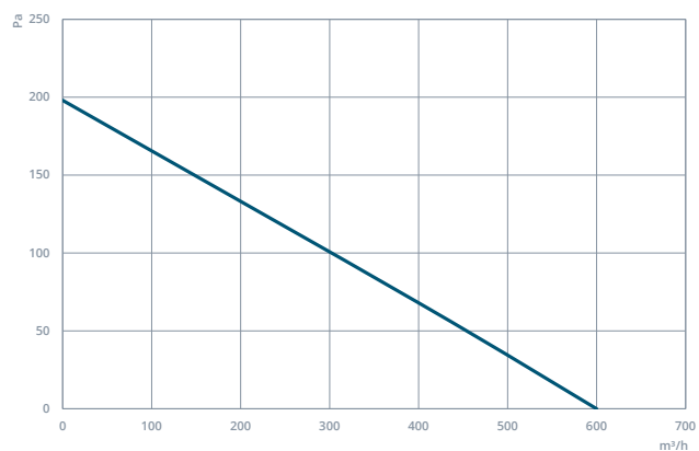
CAXIDIK 400-5-25
