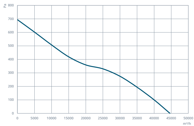
PAXI 900-5-40
