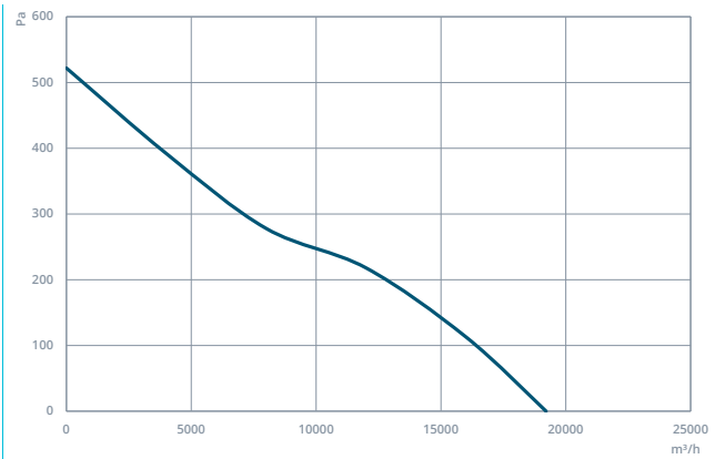
DAXI 710-5-30
