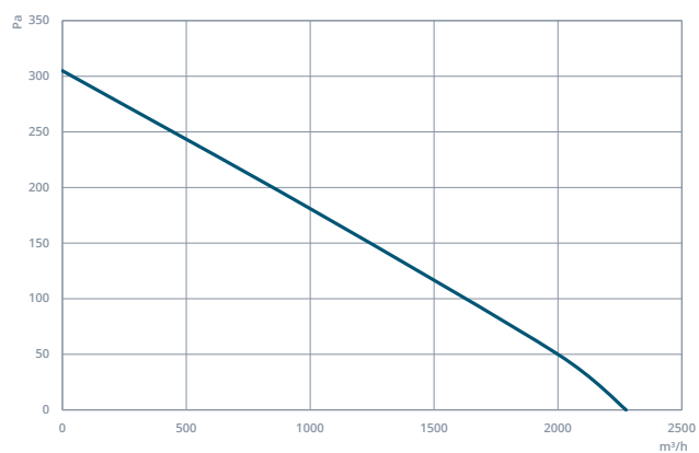
CAXIDIK 500-5-25
