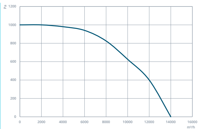
HMEF 630
