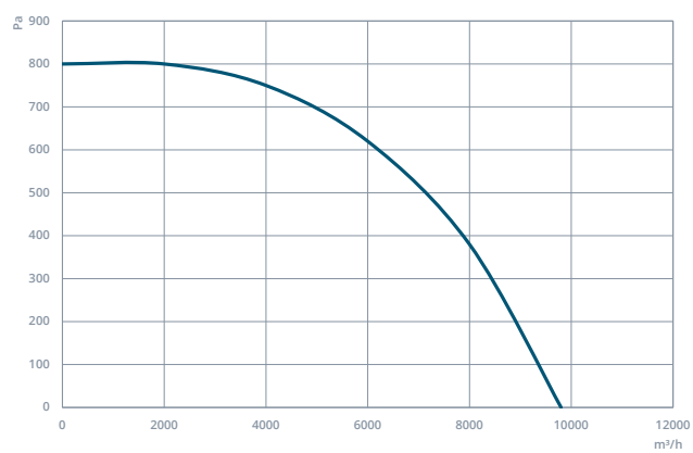
DRAD 560
