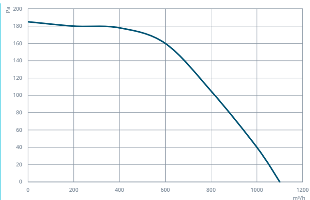
DRADIK 280
